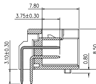
SEC A-A
