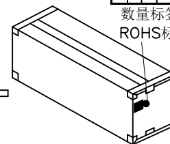
No: 5 将抽真空的产品, 放入内箱. (50管/内箱), 封箱及贴标签于内箱侧面的左上角. 内箱规格: CTN-10A (63*15*17CM)
