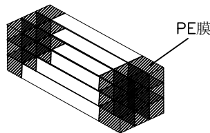
No: 3 10管为一扎(不用摆), 先用PE膜固定每扎真空管两端, 包住两端利角, 以防划破胶袋
