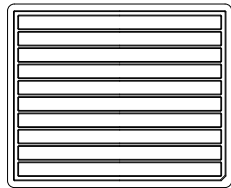
No. 1 产品装入真空盒内 SB-56AC (270*330*14.5mm) 真空盒
