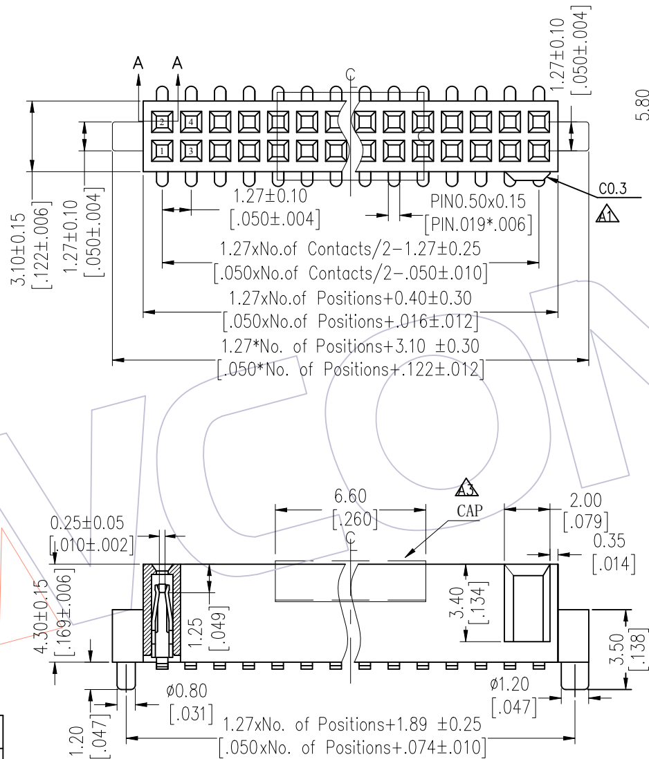
SECTION A-A
